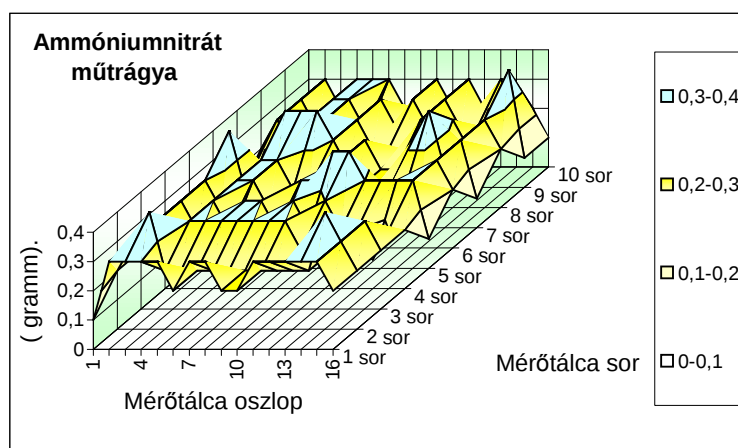
58. ábra. Teljes felületen szórás képe 150 kg/ha műtrágya mennyiség esetén
