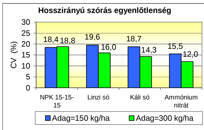
60. ábra. Hosszirányú szórás egyenlőtlenség teljes felületre szórás esetén
