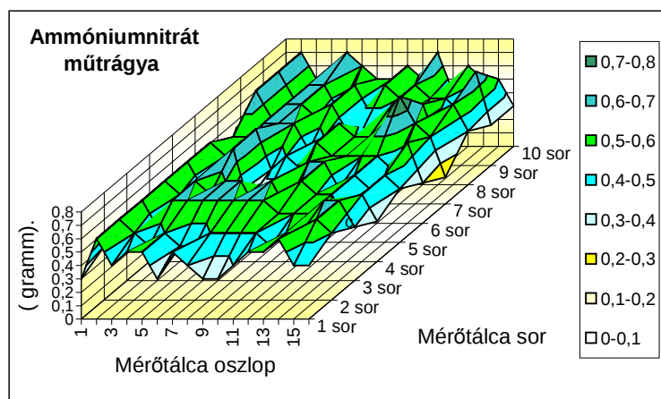
57. ábra. Teljes felületen szórás képe 300 kg/ha műtrágya mennyiség esetén
