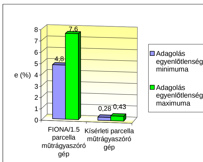
55. ábra. A FIONA/1.5 és a kísérleti műtrágyaszóró gép adagolás egyenlőtlenségének összehasonlítása NPK 15-15-15 műtrágya szórása esetén
