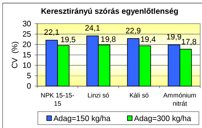
59. ábra. Keresztirányú szórás egyenlőtlenség teljes felületre szórás esetén
