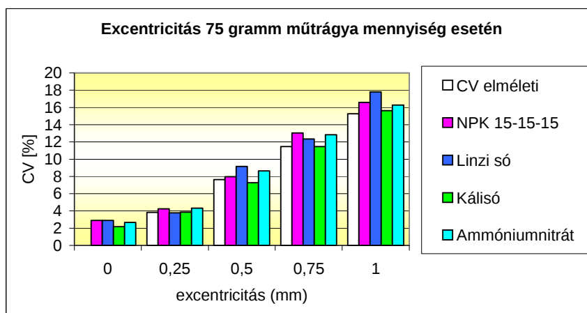
37. ábra. Az excentricitás okozta szétoztási egyenlőtlenségek
