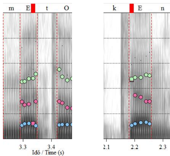
5.6. ábra. Gépi mérési hibák gépi detektálása. Formánstávolság hiba. A bal oldali ábrán az ( F_2-F_1 ) távolság, míg a jobb oldali részen az ( F_3-F_2 ) távolság túl kicsi. A függőleges tengely a frekvencia, amely 0–5000 Hz-ig jelenik meg
