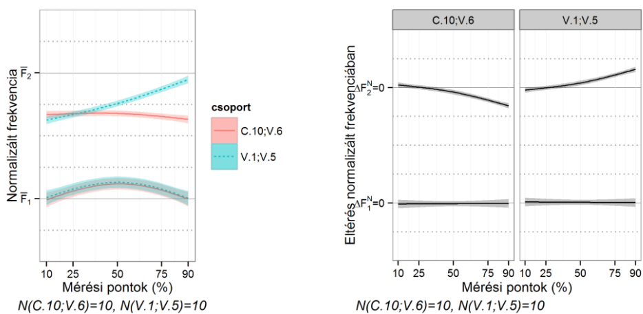
6.19. ábra. A +2. hang szignifikáns hatásának bemutatása a magánhangzó második formánsára. A bal oldali ábrán a spline-okkal modellezett jellemző görbék láthatók a két csoportban. A jelmagyarázat a -2. és +2. hang kategóriáját tartalmazza (C.10;V.6=[vɔho]; V.1;V.5=[vɔhi]). A jobb oldali ábrán a csoport és interakciós hatás együttesen jelenik meg
