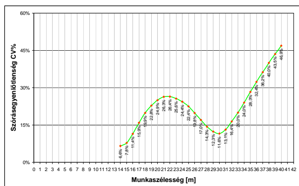
32. ábra. Szórás kép előre állított lapátokkal
