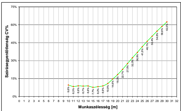
26. ábra. Kálicsival végzett mérés
