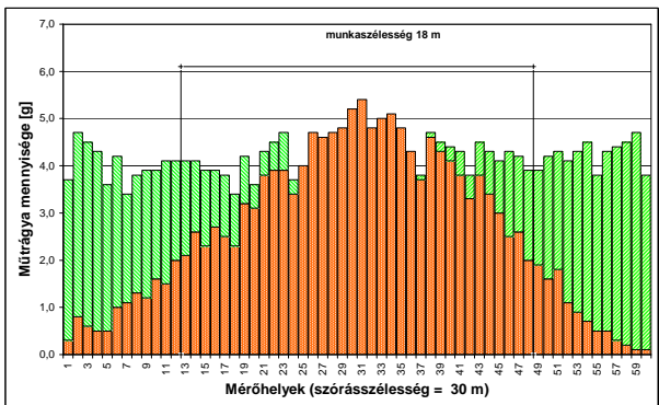
24. ábra. Mérés B2 adagolási helytel
