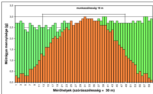
23. ábra. Mérés B3 adagolási helytel
