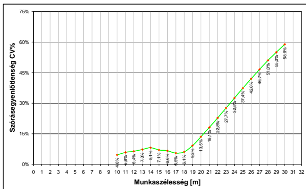
25. ábra. Ammóniumnitráttal végzett mérés
