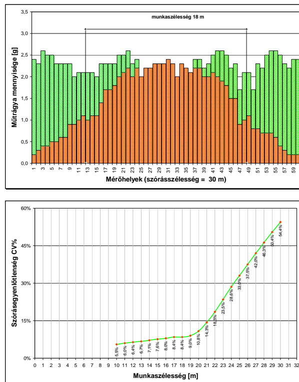
37. ábra. Mérés 106°-os lapáttal
