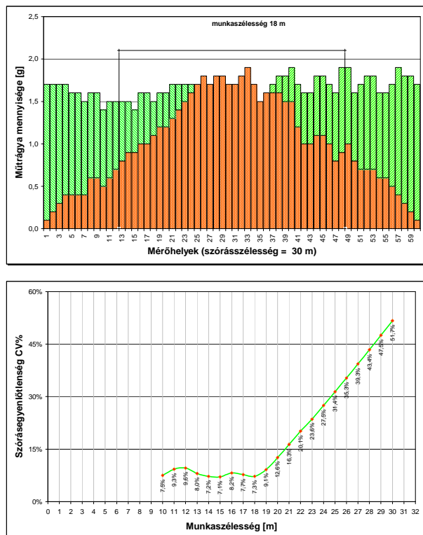
36. ábra. Mérés 90°-os lapáttal
