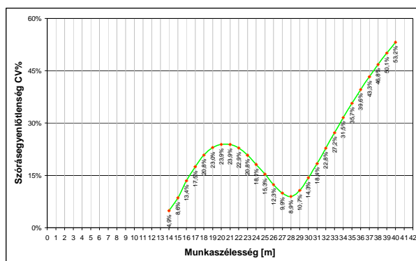
33. ábra. Szórás kép hátra állított lapátokkal
