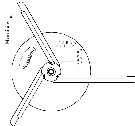
20. ábra. A röpitőtárcsa felületéhez viszonyított adagolási helyek
