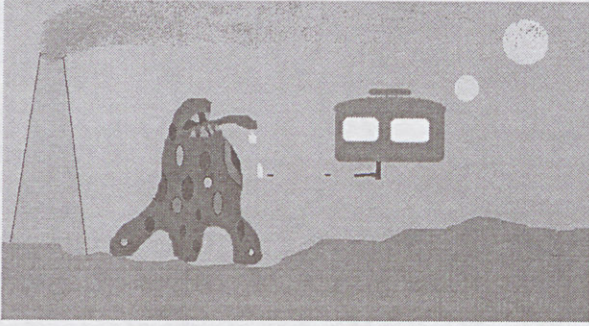
Half-life
