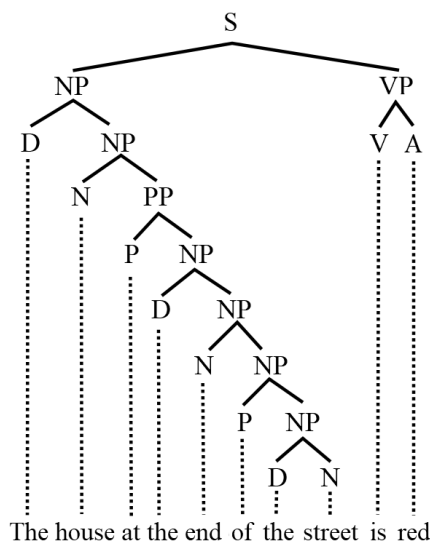
10. ábra. Frázisstruktúra-nyelvtan (forrás: Tjo3ya – Own work, CC BY-SA 3.0, https://commons.wikimedia.org/w/index.php?curid=18436919 ). A szerkezet kontextusfüggetlen, hiszen rajta az ún. frázisok (más néven: kifejezések; lényegében: egyszerűbb-komplexebb összetevők) hierarchikusan helyezkednek el.
