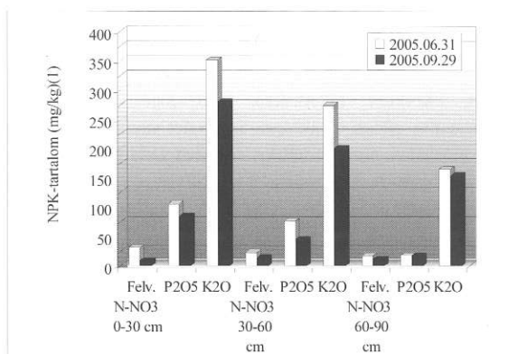
7. ábra: Az NPK-tartalom változása 2005-ben szolonyeces réti talajon
