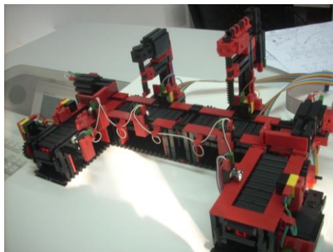
3.4. ábra: Gyártócella maróval és fűrővel
