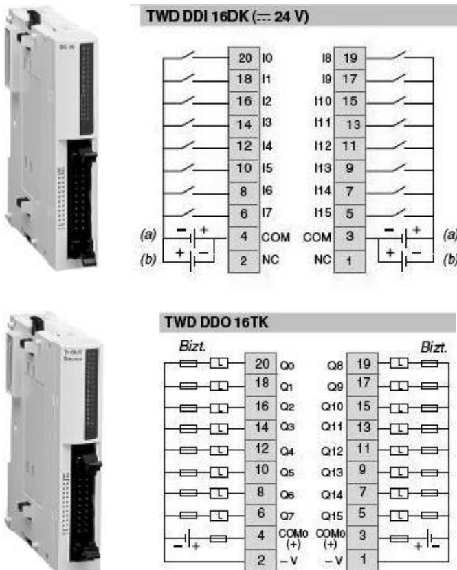
2.11 ábra: I/O bővítőegységek
