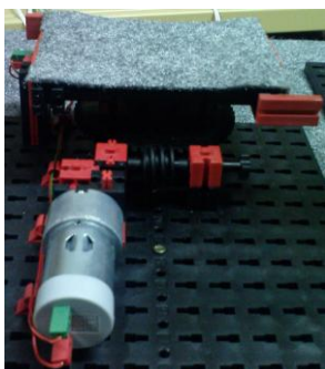
3.17. ábra: Paletta 2
