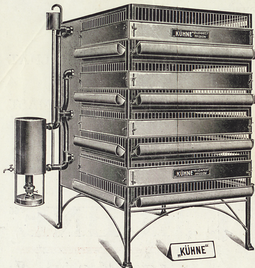
Melegvízfűtéses csibenevelő- és hizlaló ketrec 500 csibe részére.
