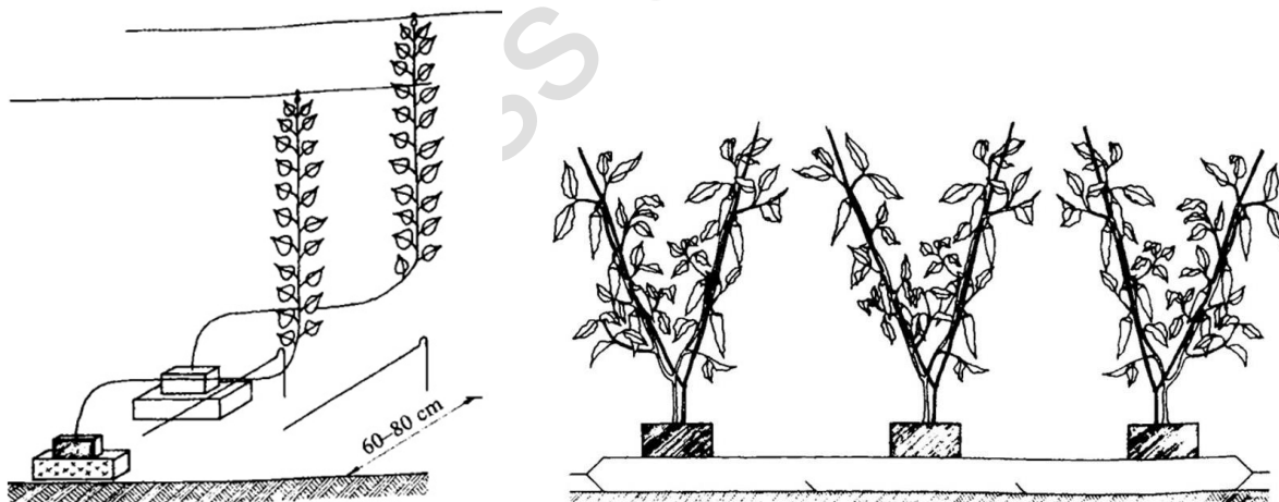
14. ábra. A főszár terheléses metszés és a kötözés vázlatja paprika kőgyapotos termesztésénél (Forrás: Slezák és Terbe, 2008)
