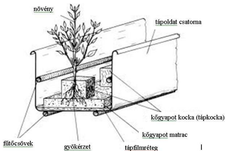
4. ábra. Az NFT zöldségtermesztési módszer vázlatja (Forrás: Balázs, 1994)
