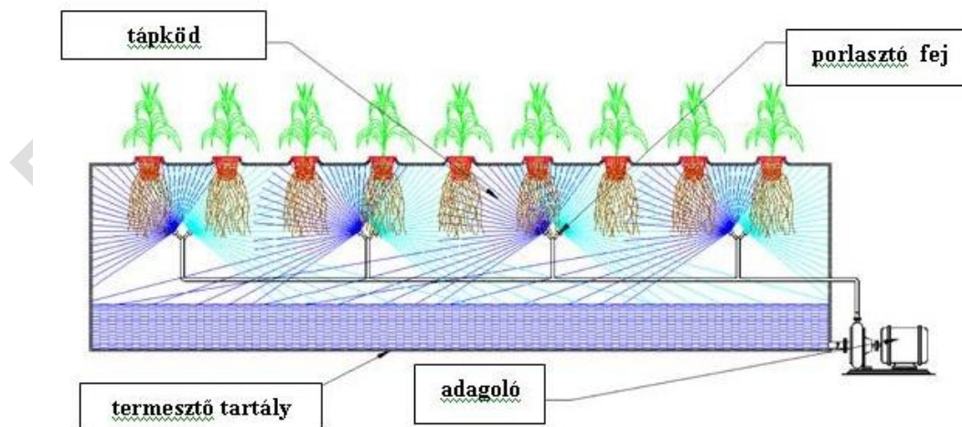
7. ábra. Aeropóniás rendszer (Forrás: Internet 1)
