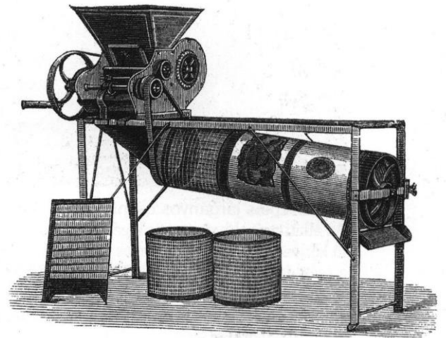
10. kép. Mayer-féle konkolyozó.
