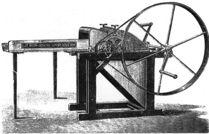
9. kép. Kézi hajtású cséplőgép 1896-ból.
