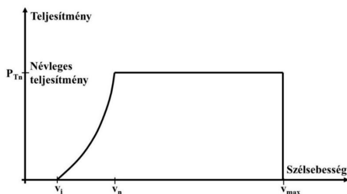
32. ábra. A szélerőművek jellemző szélesebbesség-teljesítmény görbéje
